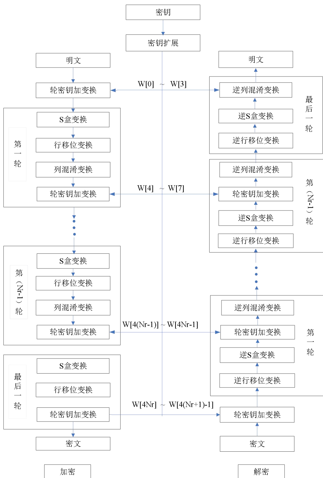
图 3 AES 加/解密过程图
